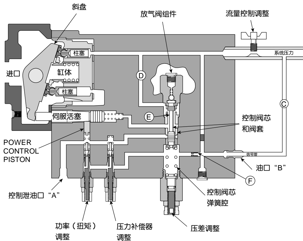
控制选项 — ‘C’
