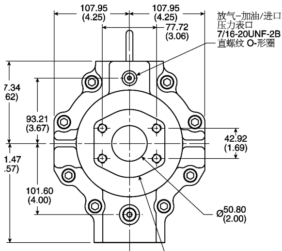
后进油口 (进口选项 "省略") 见油口尺寸表
